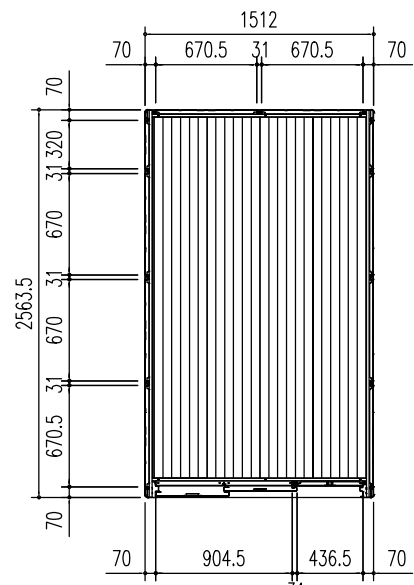
平面図 (S=1/50)
