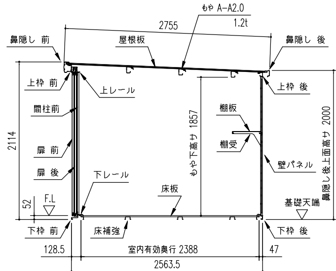
短計図 (S=1/50)
