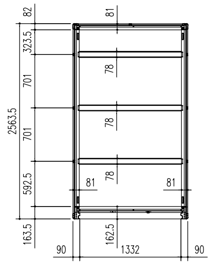
床伏図 (S=1/50)
