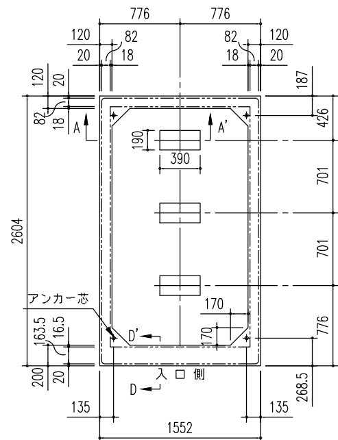
布基礎伏図 (S=1/50)
