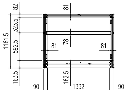
床伏図 (S=1/50)
