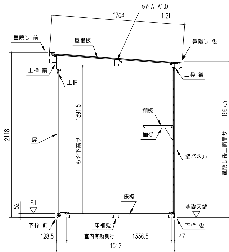
矩計図 (S=1/30)
