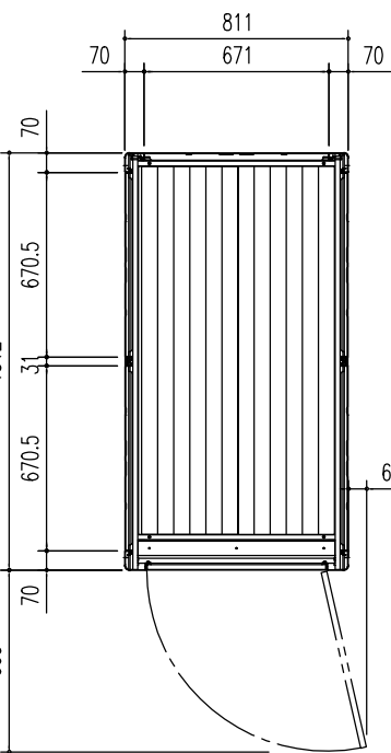
平面図 (S=1/30)
