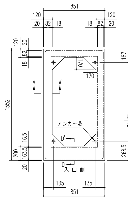
布基礎伏図 (S=1/30)
