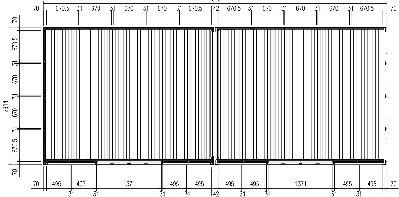
平面図 (S = 1/50)
