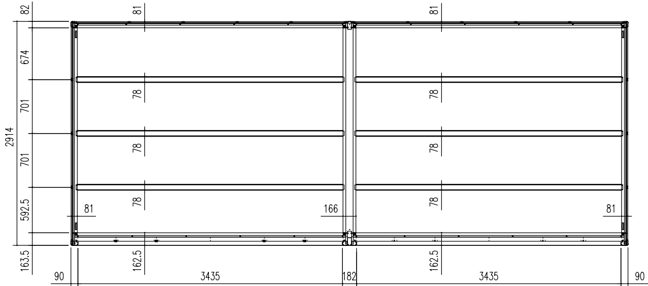
床伏図 (S = 1/50)
