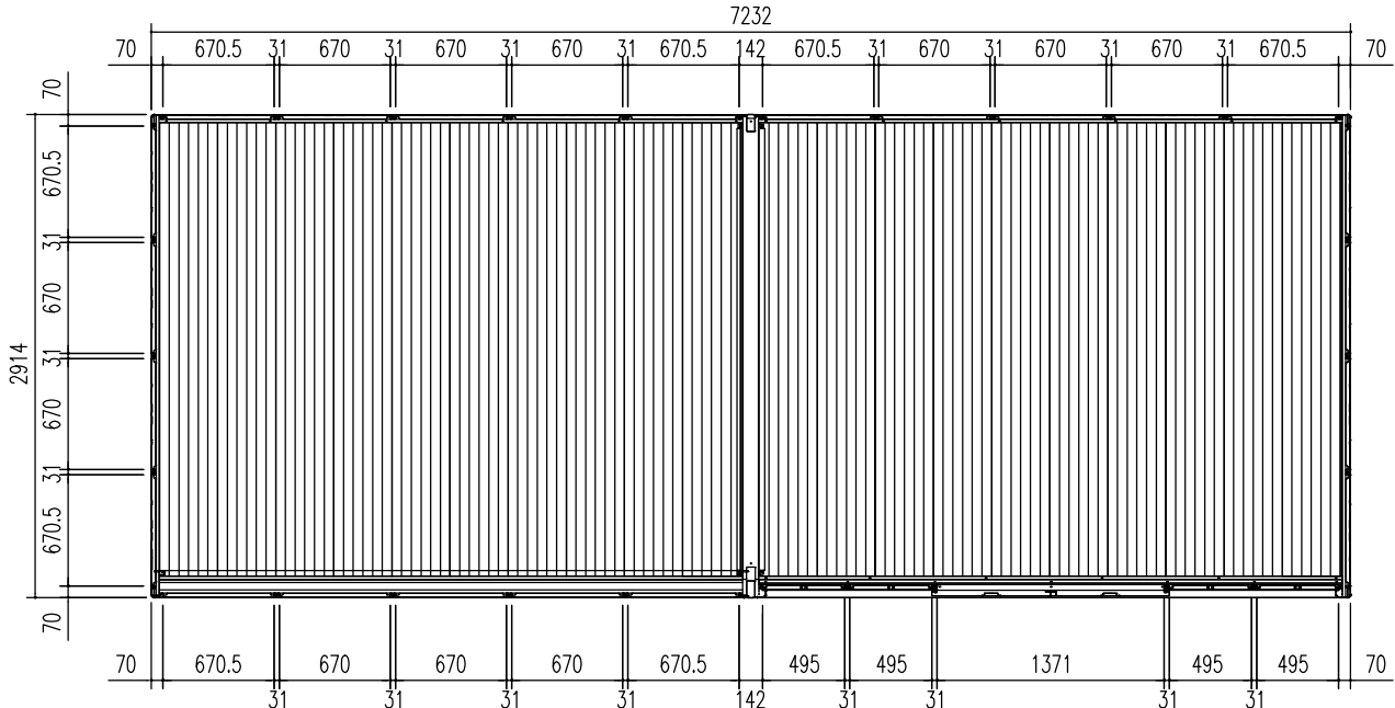
平面図 (S = 1/50)
