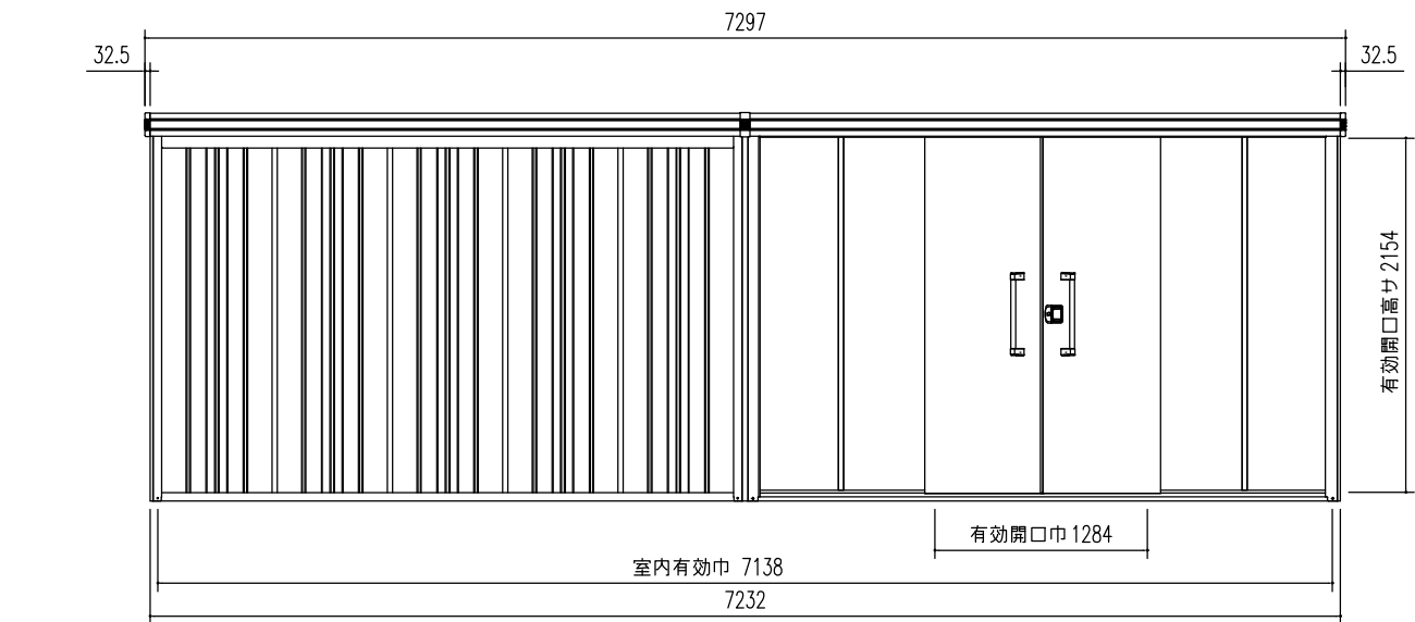
正面立面図 (S = 1/50)
