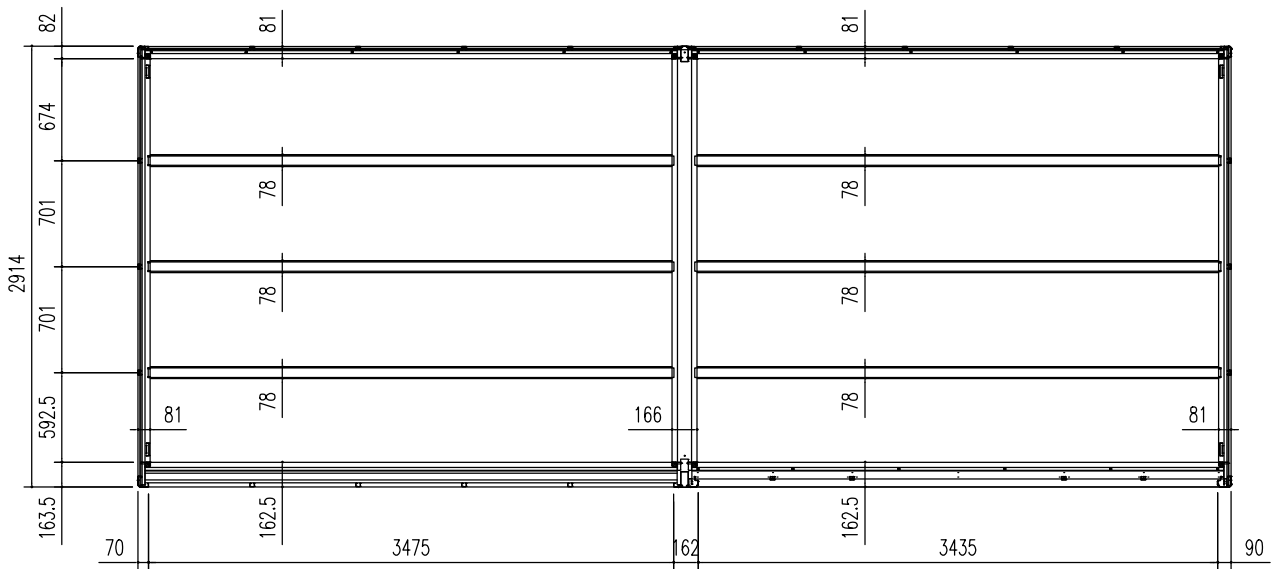
床伏図 (S = 1/50)
