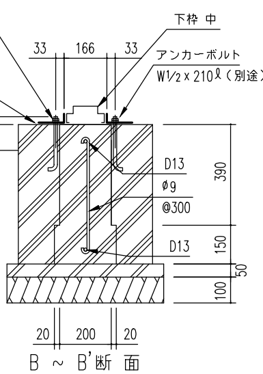
布基礎断面図例 (S=1/20)
