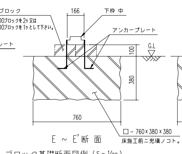
ブロック基礎断面図例 (S=1/20)
