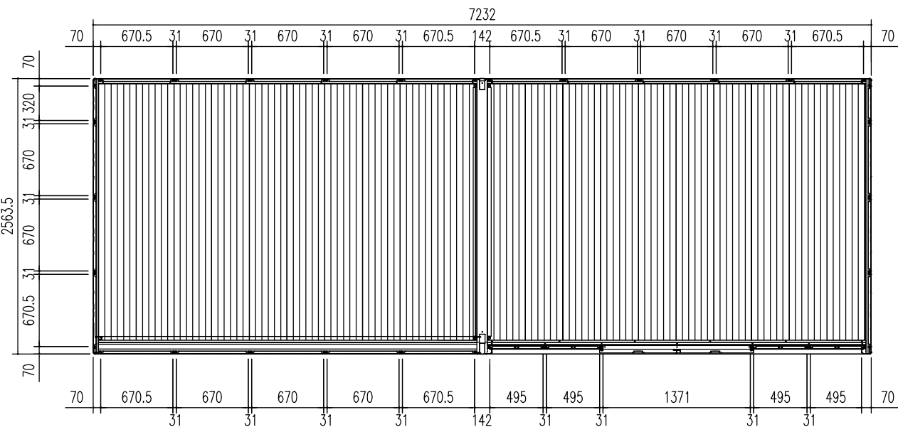
平面図 (S = 1/50)
