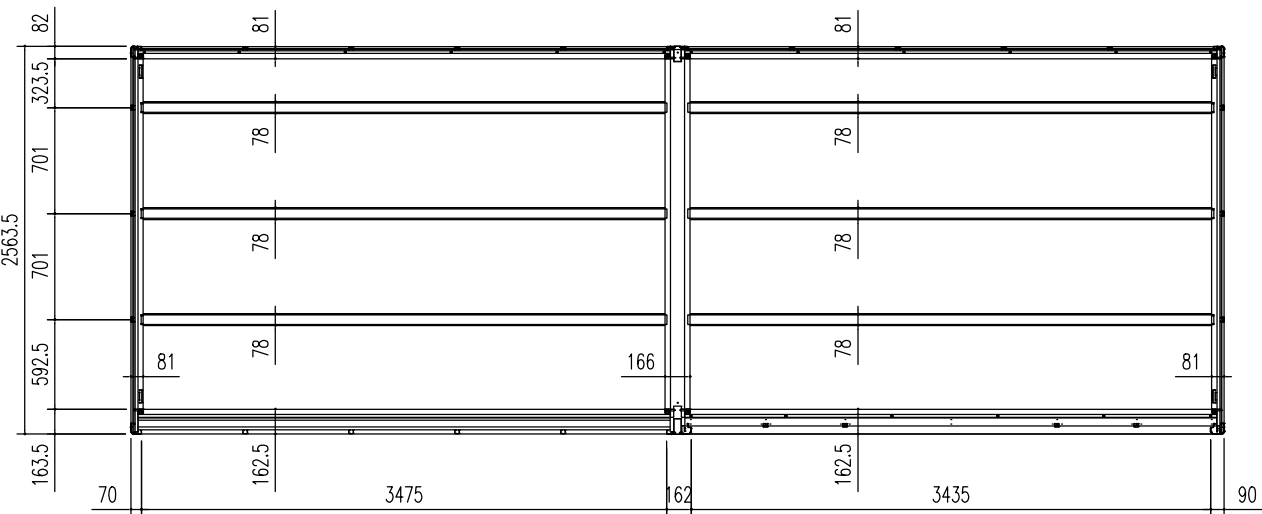
床伏図 (S = 1/50)
