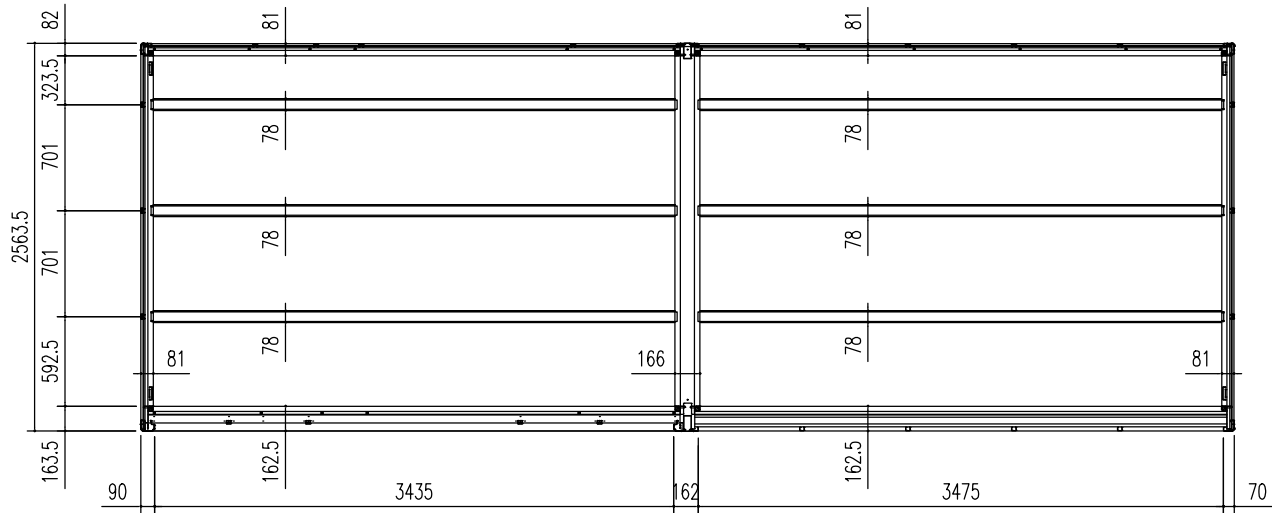
床伏図 (S = 1/50)
