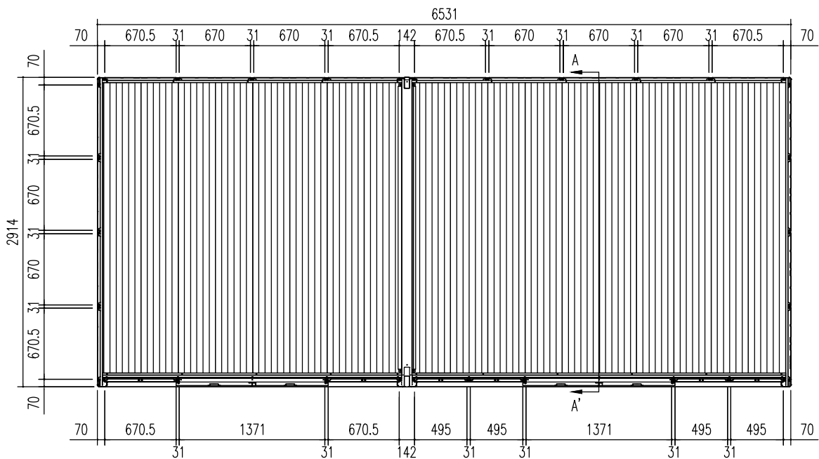
平面図 (S=1/50)
