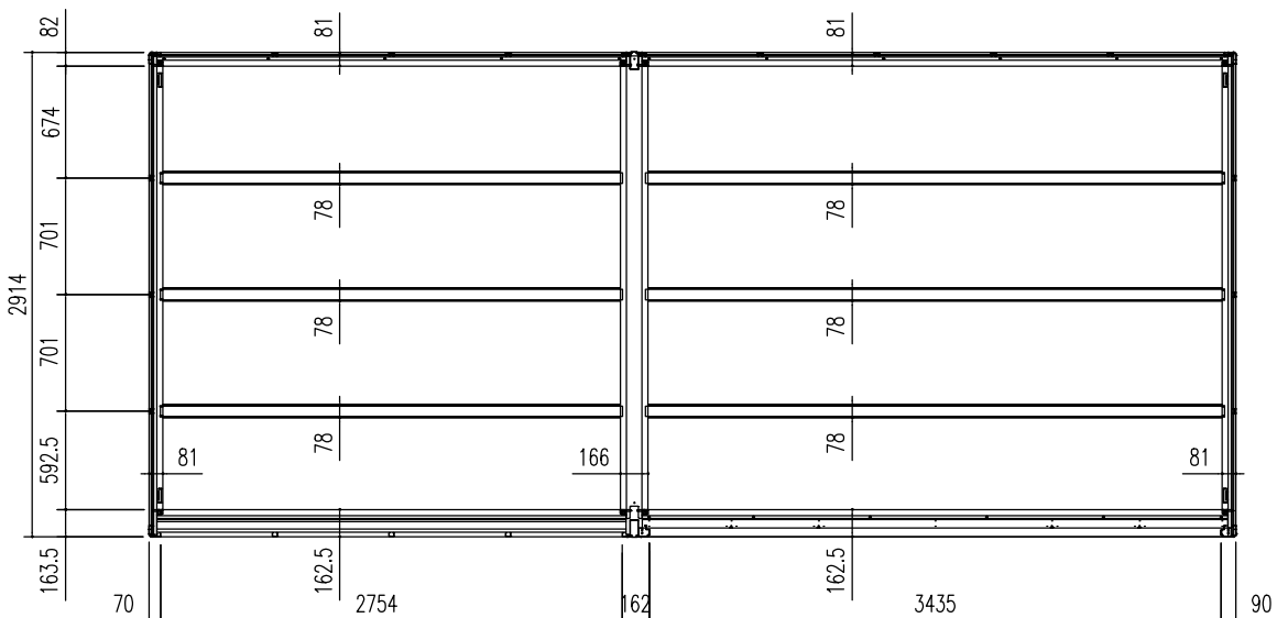
床伏図 (S = 1/50)
