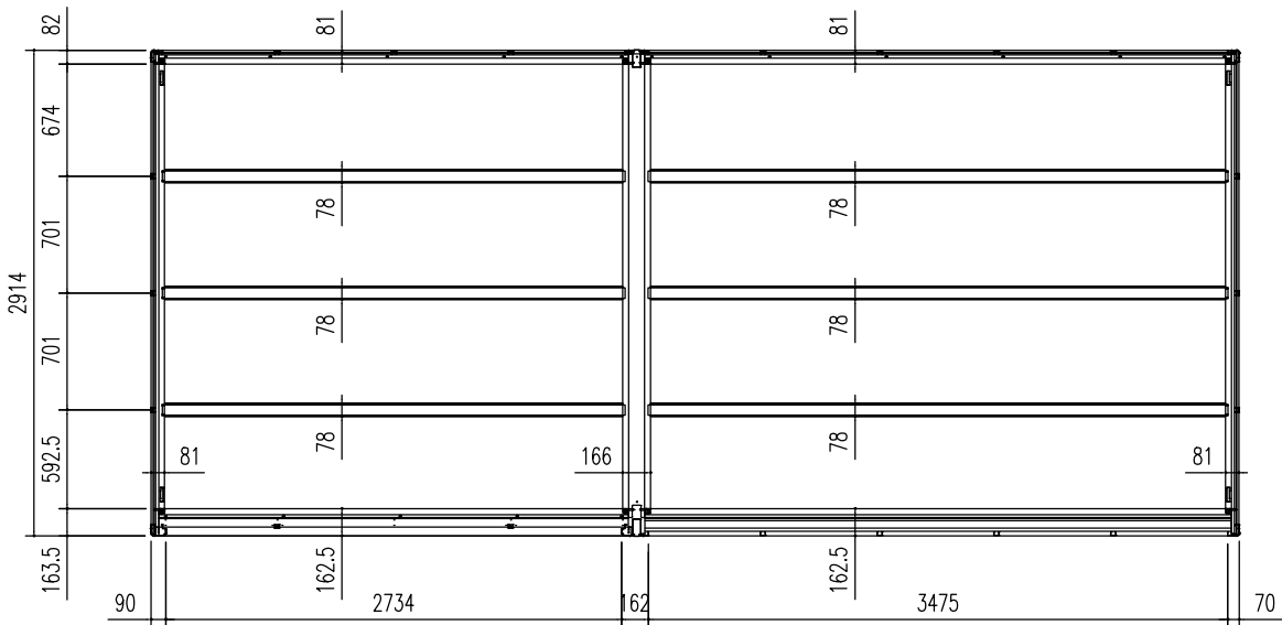
床伏図 (S = 1/50)
