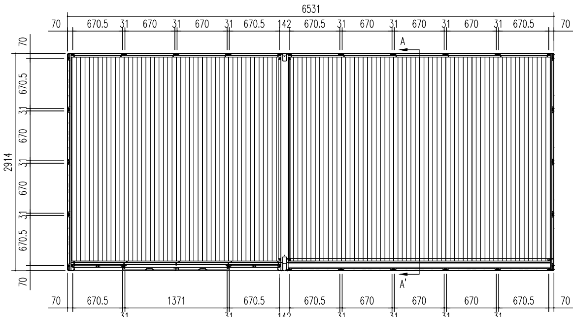
平面図 (S = 1/50)
