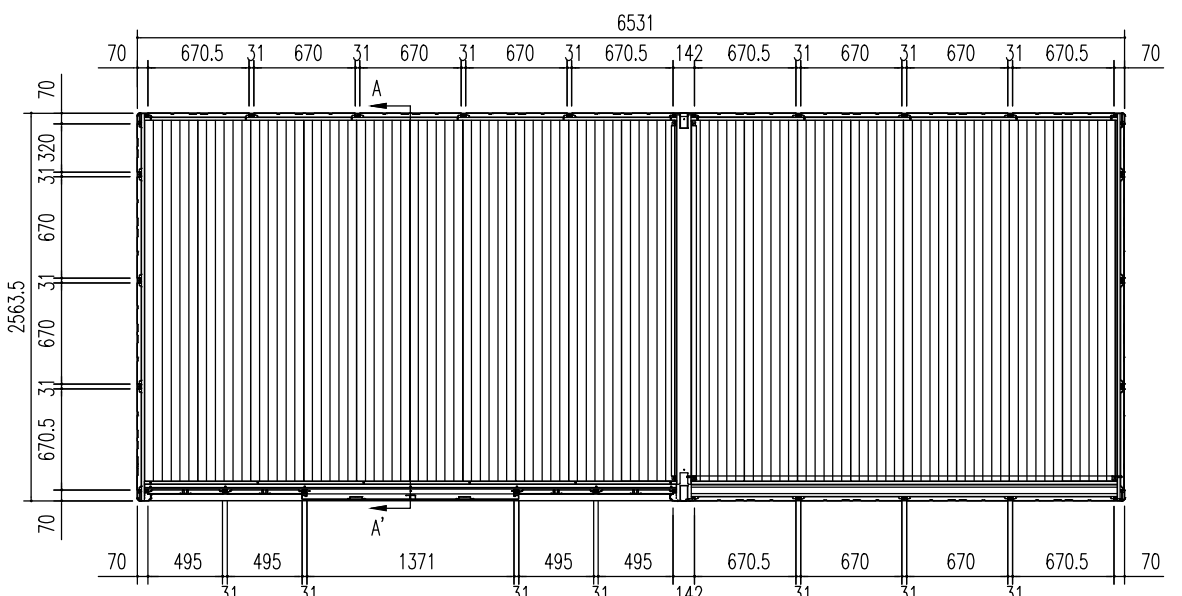
平面図 (S = 1/50)
