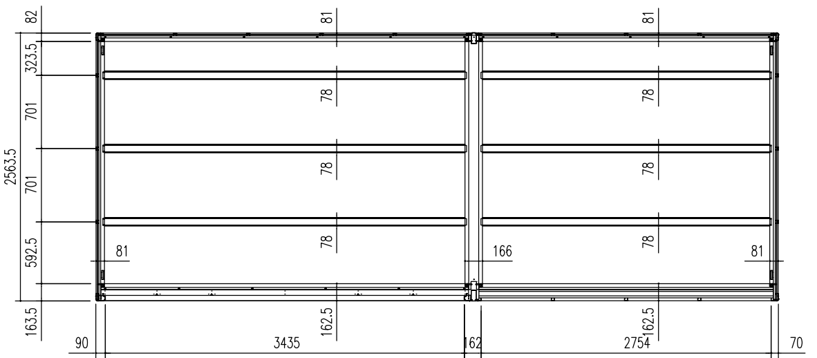
床伏図 (S = 1/50)
