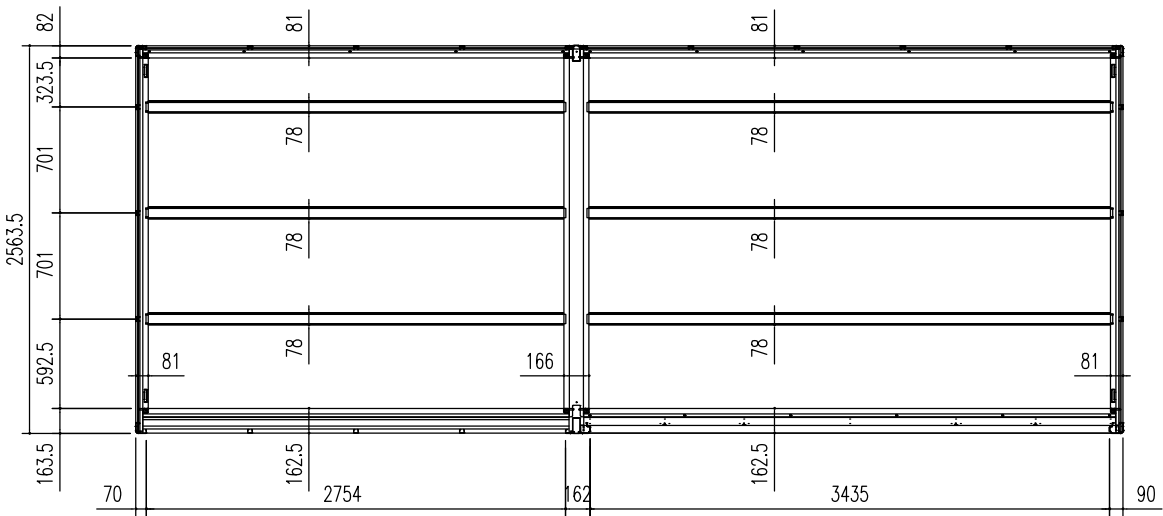
床伏図 (S = 1/50)
