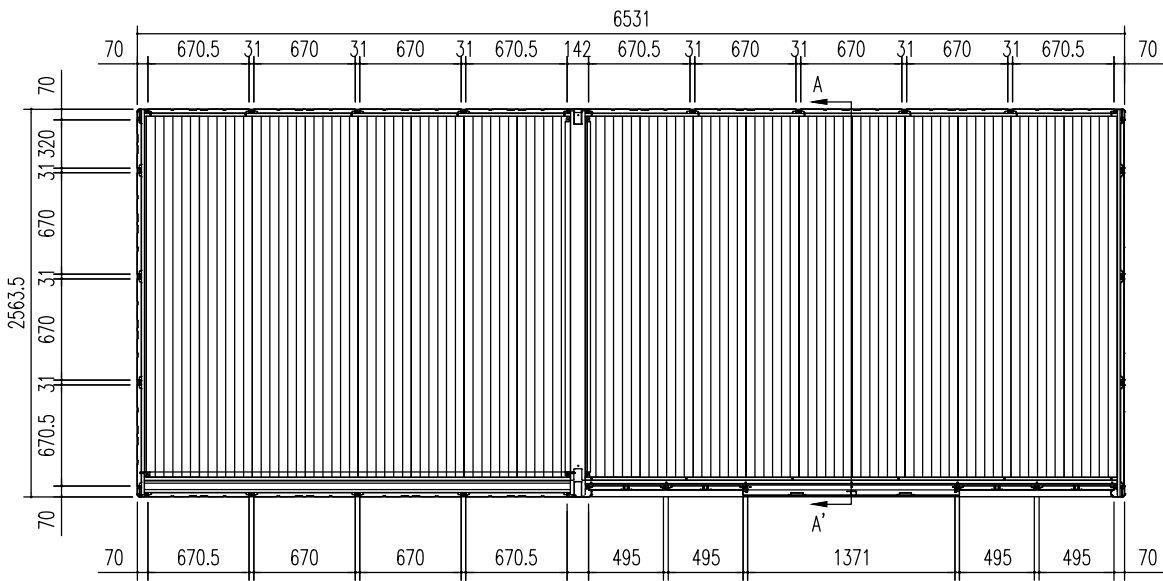
平面図 (S = 1/50)
