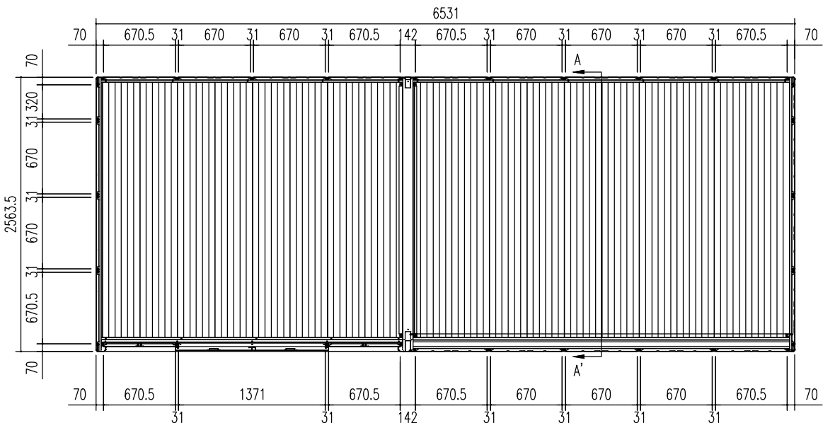
平面図 (S = 1/50)
