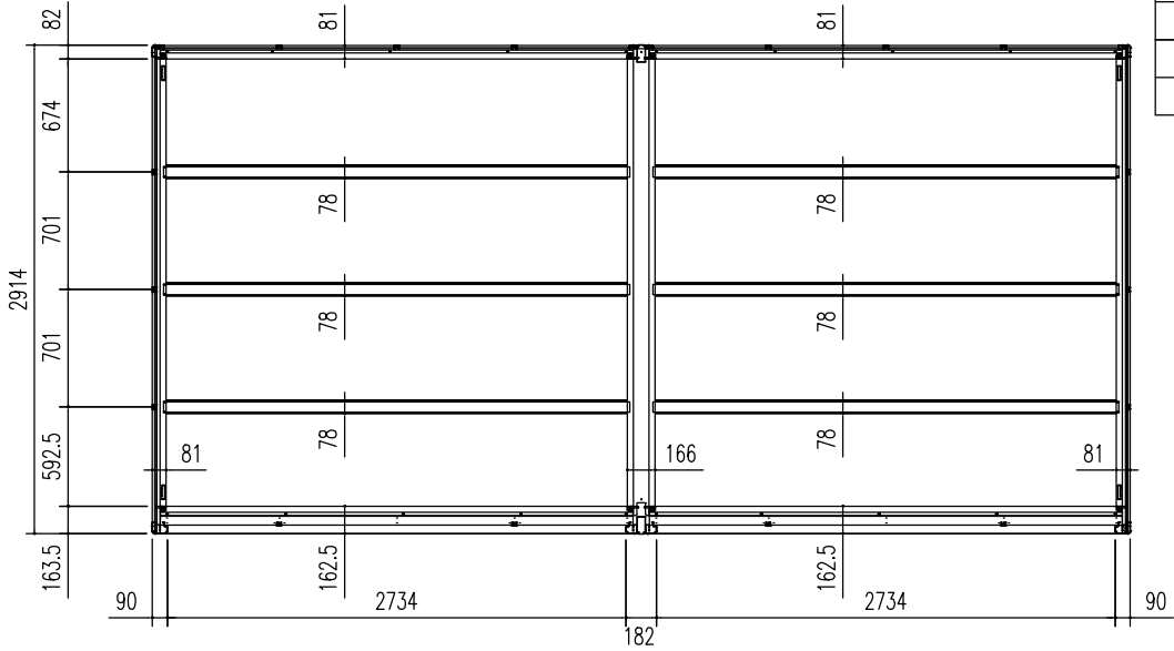
床伏図 (S = 1/50)
