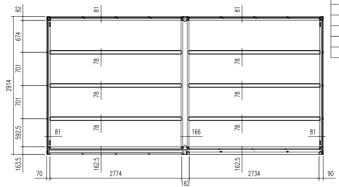
床伏図 (S=1/50)
