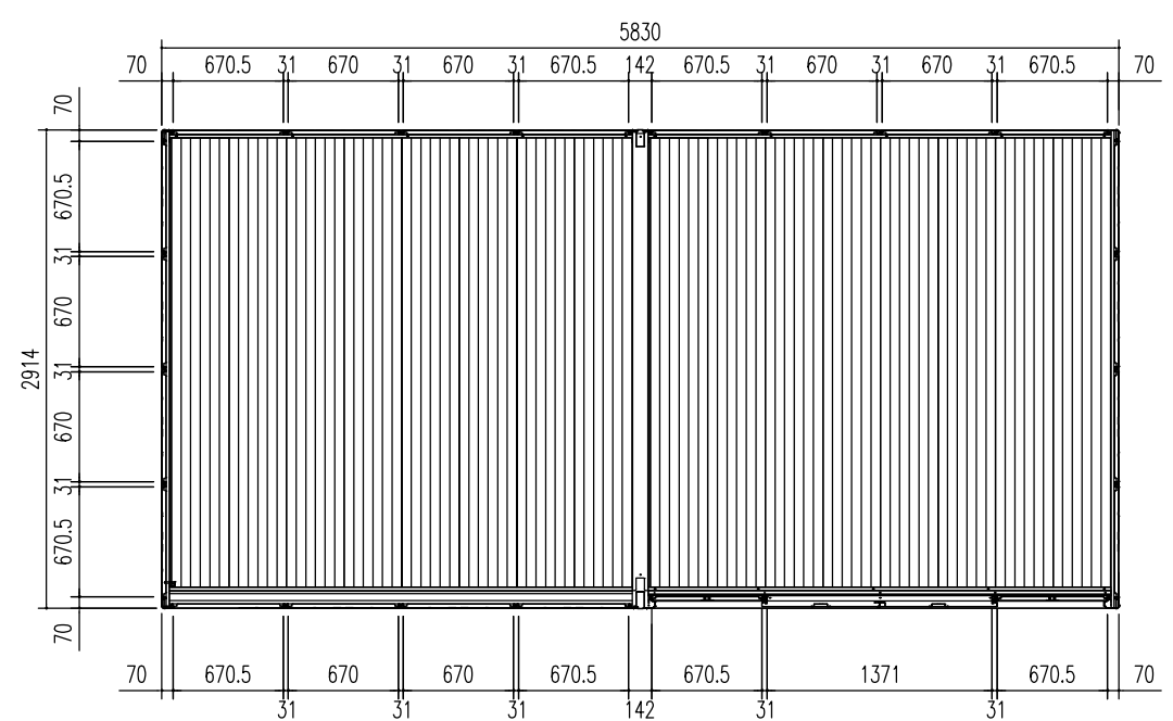
平面図 (S=1/50)
