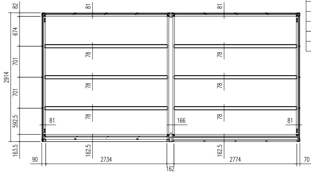
床伏図 (S=1/50)
