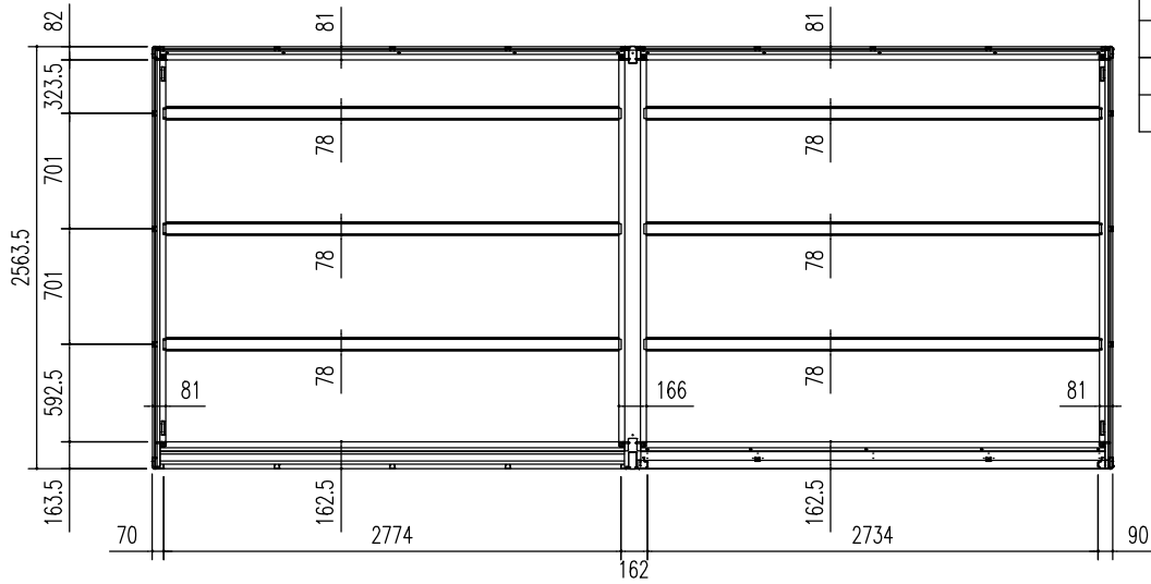
床伏図 (S=1/50)
