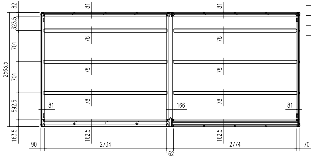
床伏図 (S=1/50)
