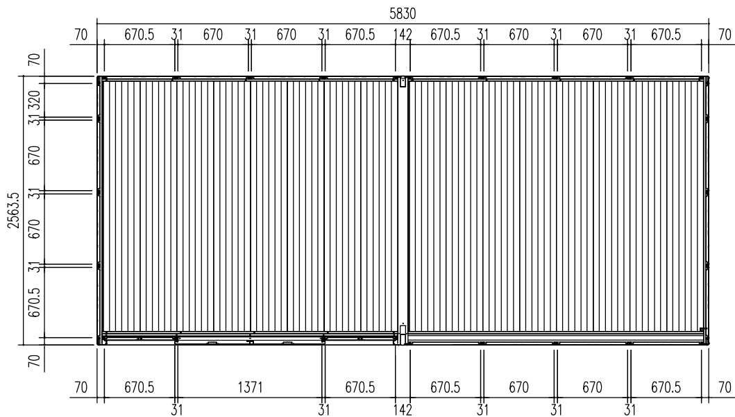
平面図 (S=1/50)
