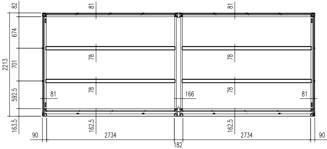
床伏図 (S=1/50)
