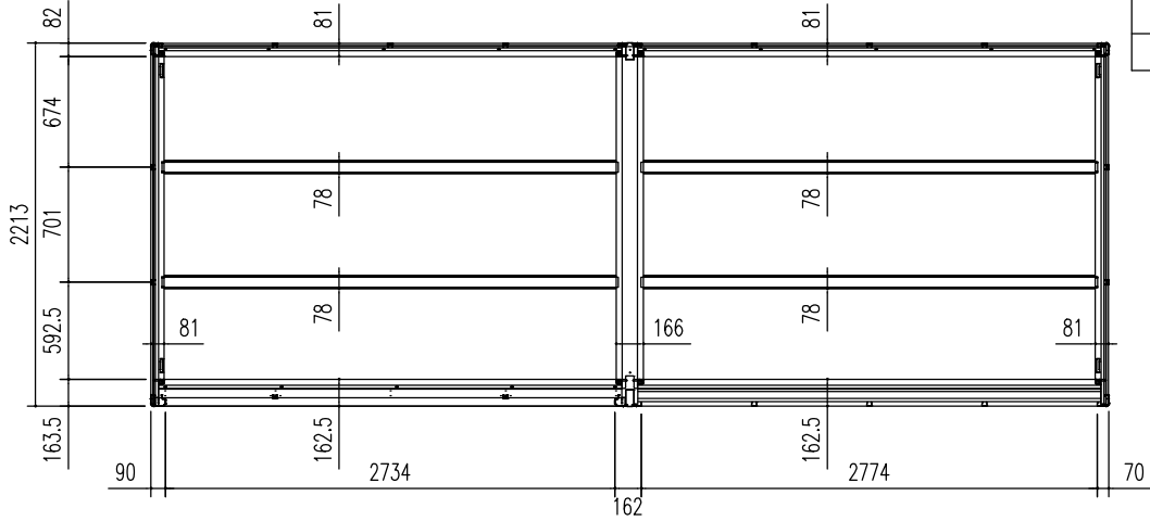
床伏図 (S=1/50)
