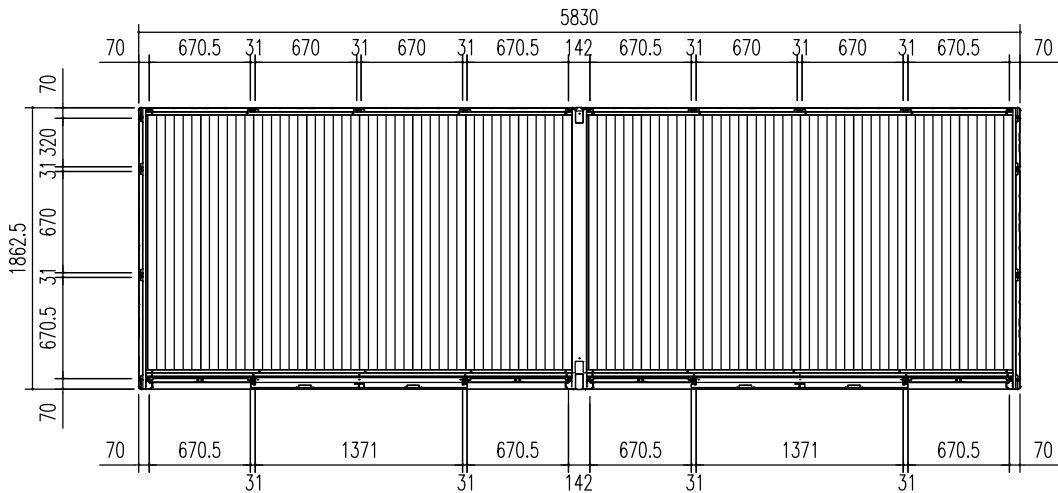
平面図 (S=1/50)
