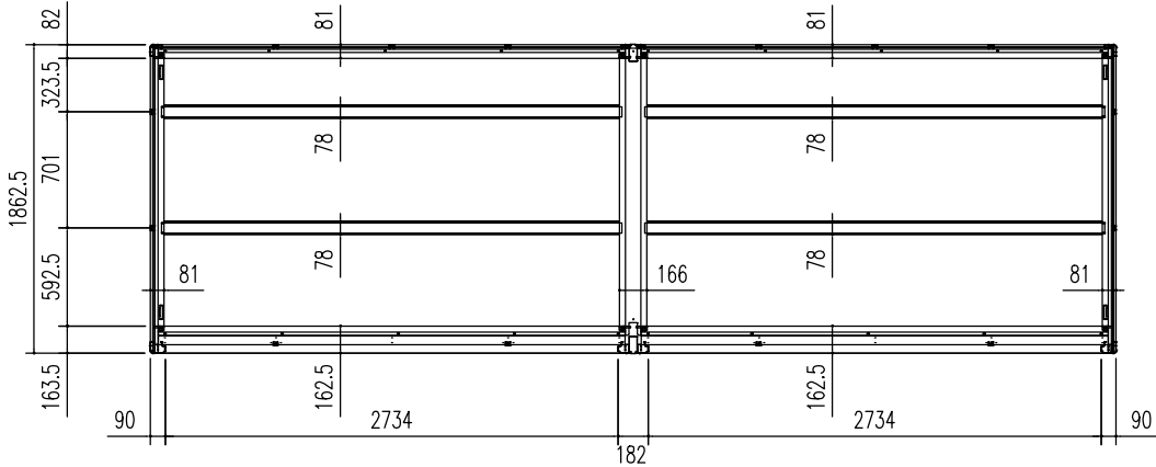
床伏図 (S=1/50)
