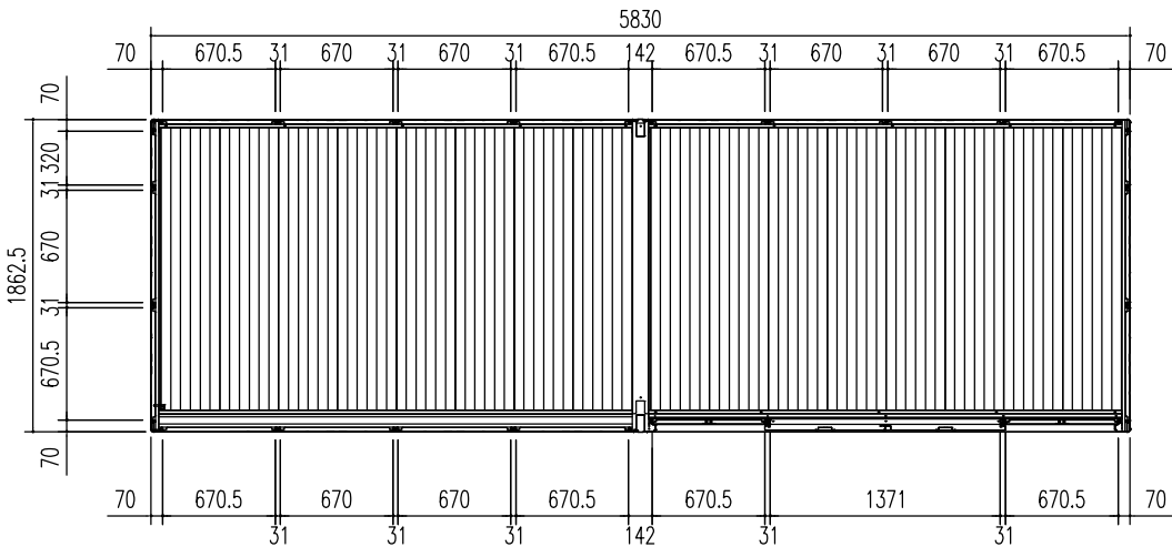
平面図 (S=1/50)
