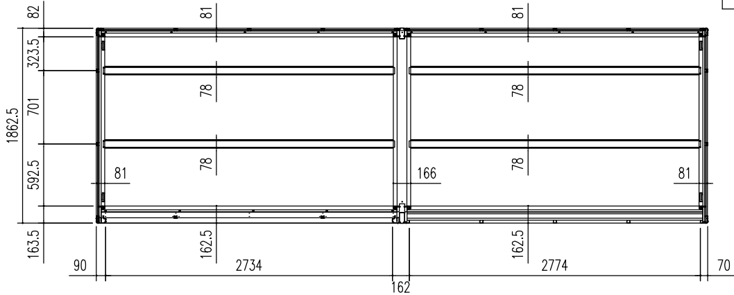
床伏図 (S=1/50)
