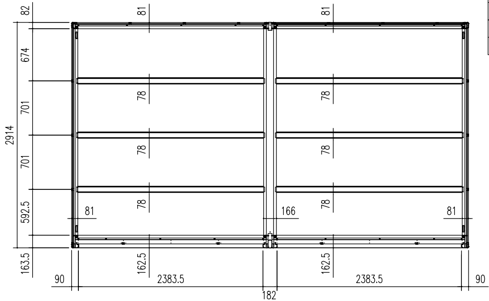
床伏図 (S=1/50)
