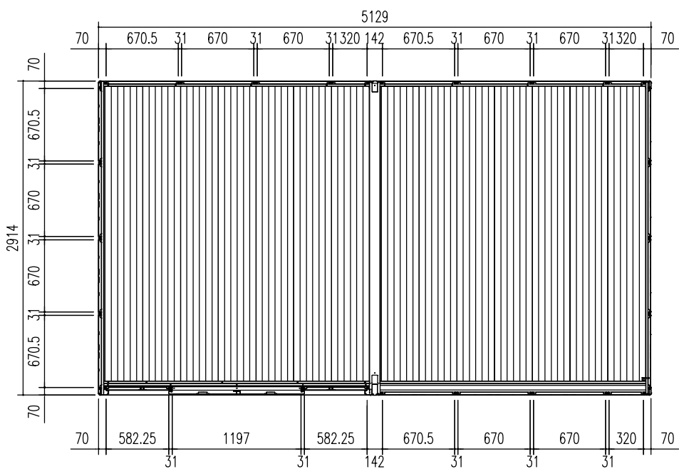
平面図 (S=1/50)
