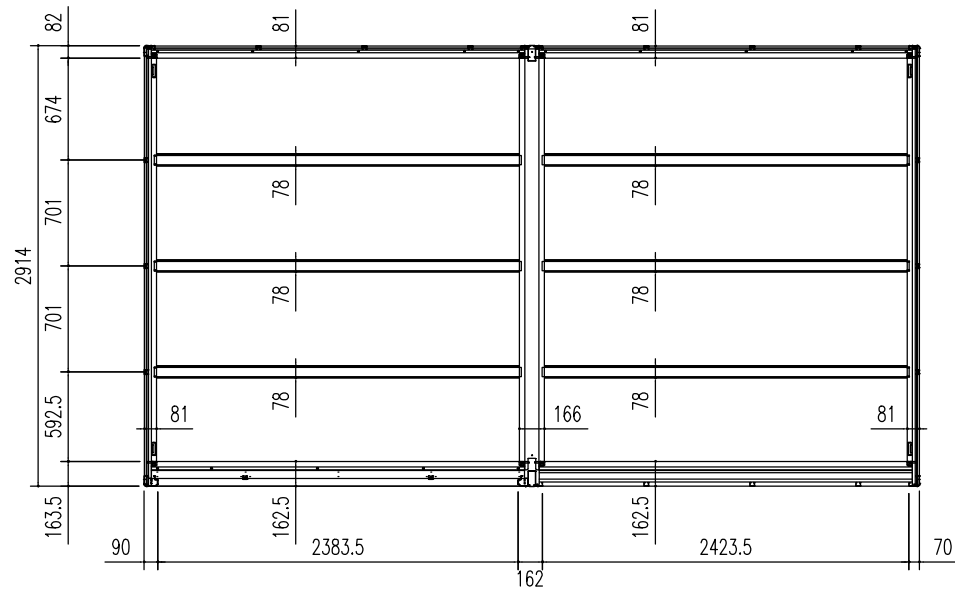
床伏図 (S=1/50)
