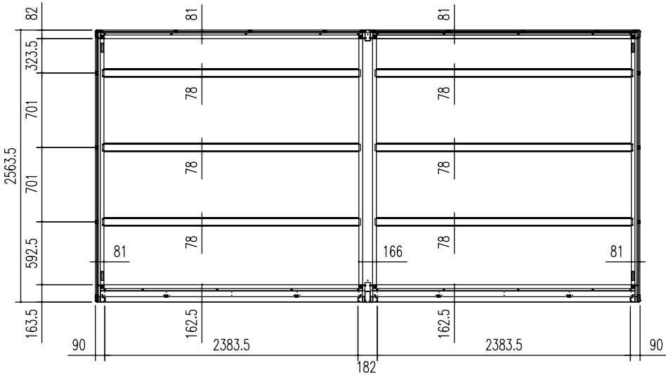
床伏図 (S=1/50)
