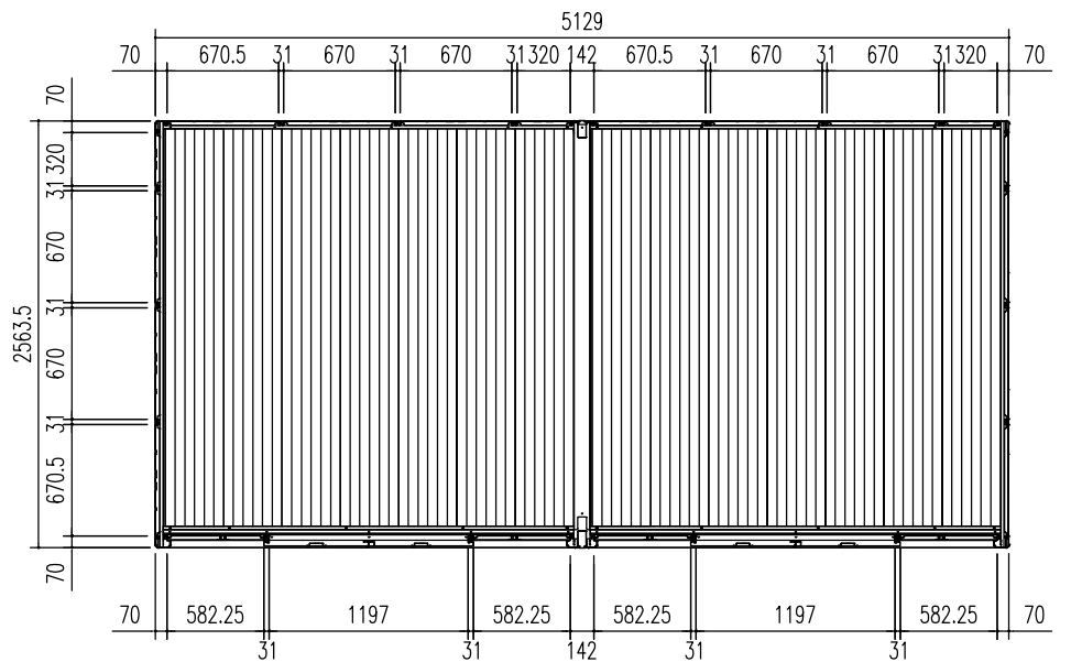
平面図 (S=1/50)
