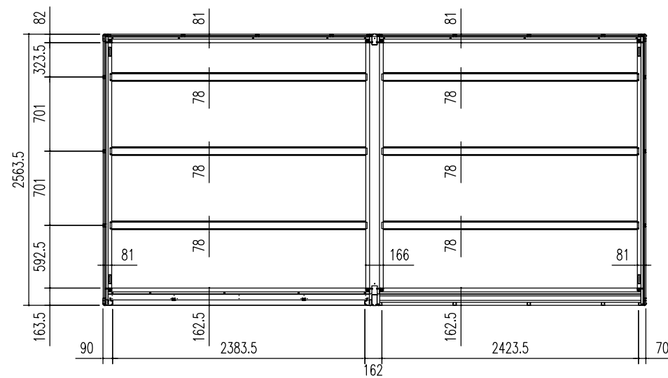
床伏図 (S=1/50)
