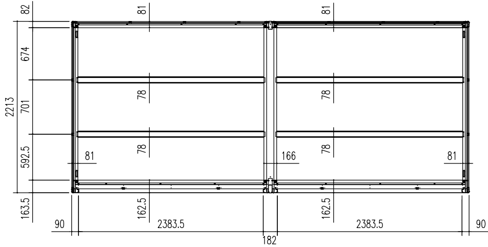
床伏図 (S=1/50)
