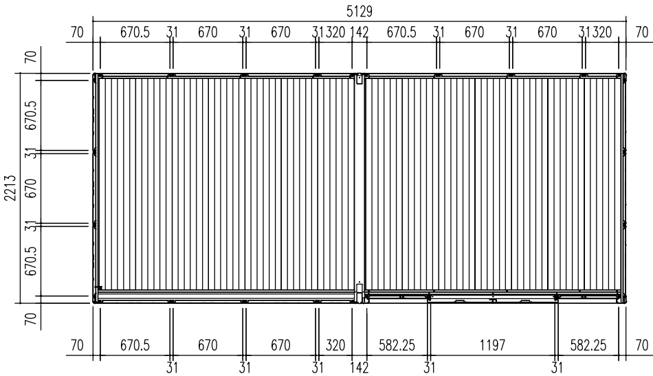
平面図 (S=1/50)
