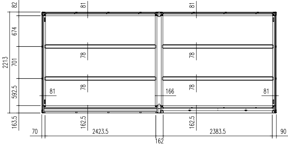
床伏図 (S=1/50)
