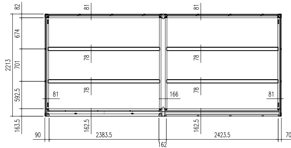
床伏図 (S=1/50)
