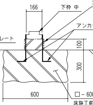
E ~ E' 断面 (内アンカー用)
