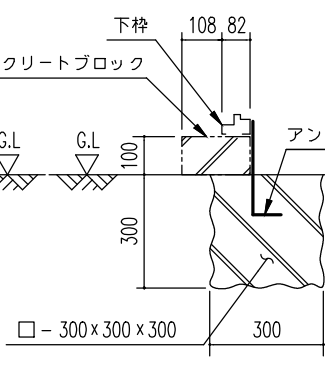
D ~ D' 断面 (外アンカー用)
