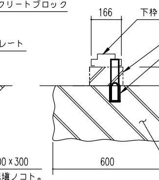
F ~ F' 断面 (外アンカー用)
