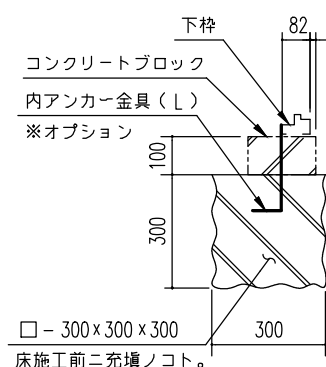
C ~ C' 断面 (内アンカー用)
