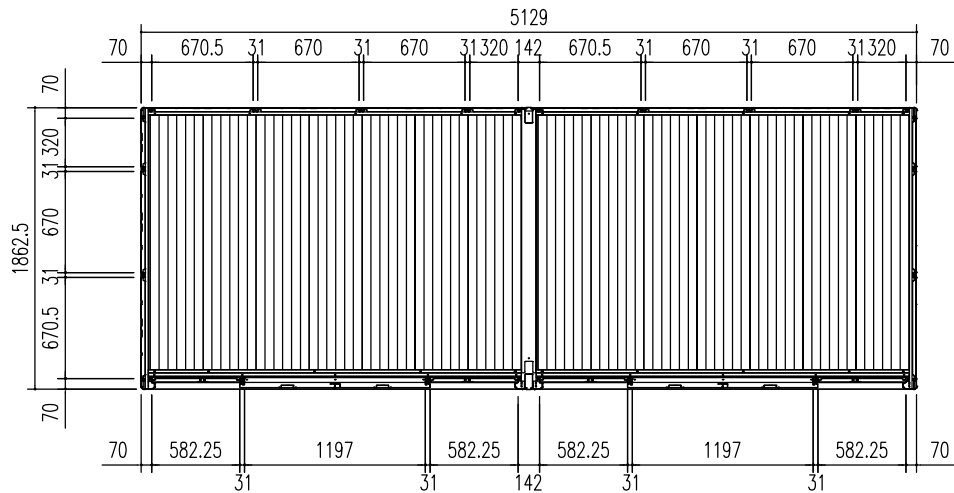
平面図 (S=1/50)
