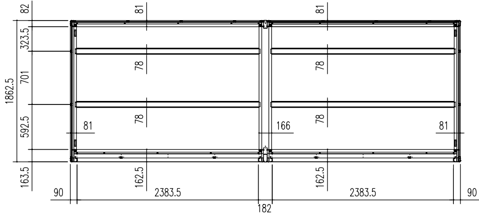
床伏図 (S=1/50)
