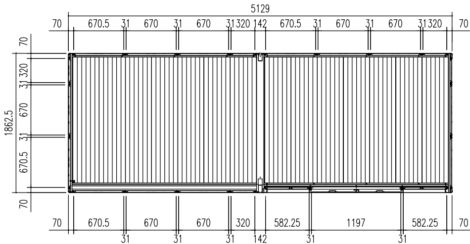
平面図 (S=1/50)
