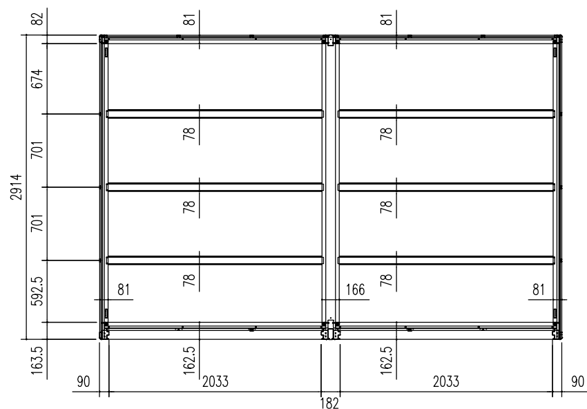
床伏図 (S=1/50)
