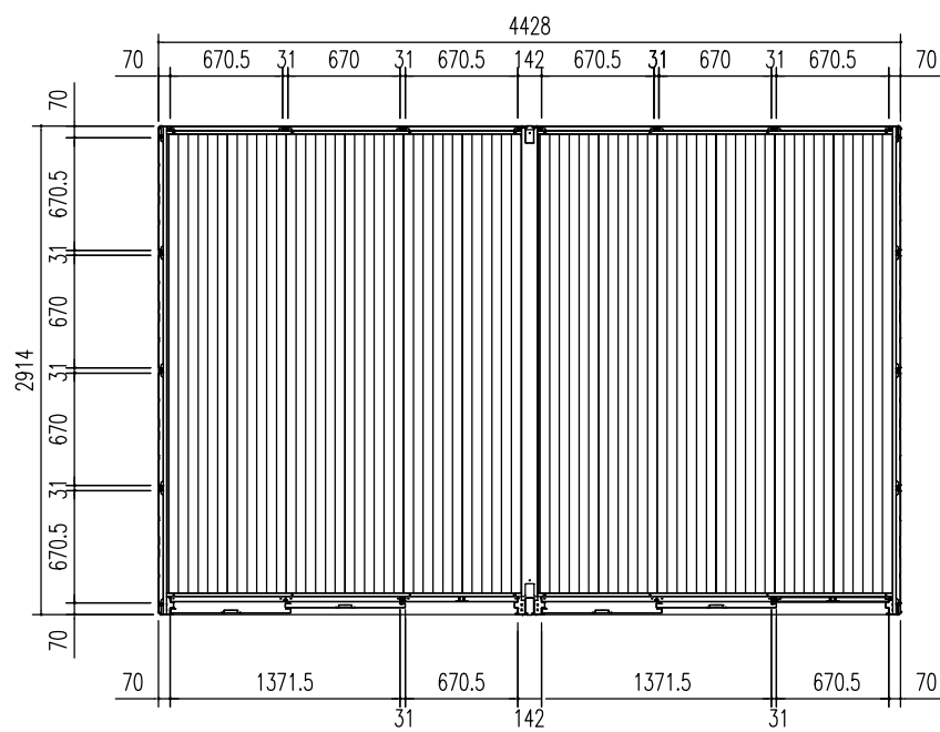
平面図 (S=1/50)
