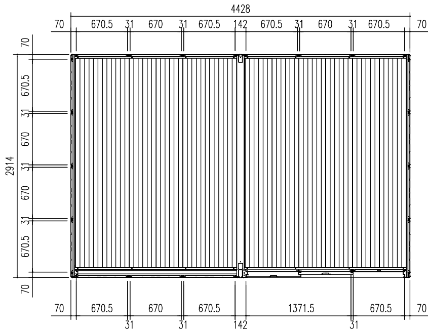
平面図 (S=1/50)
