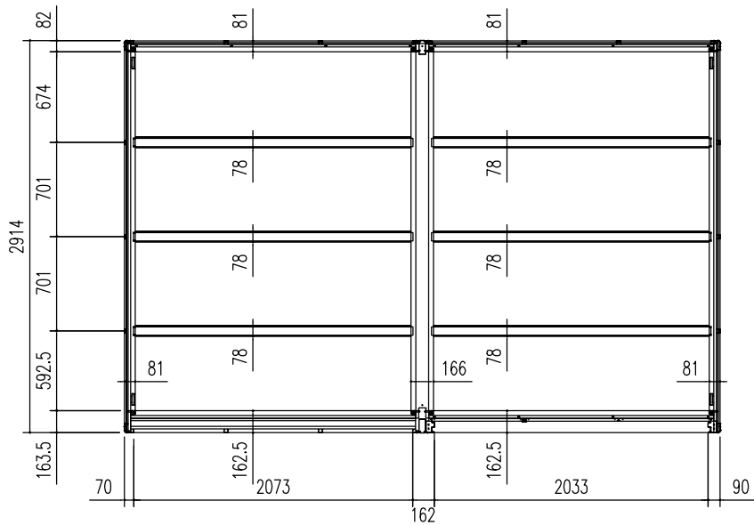
床伏図 (S=1/50)
