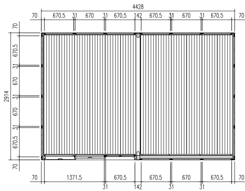
平面図 (S=1/50)
