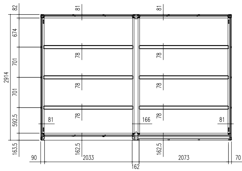
床伏図 (S=1/50)
