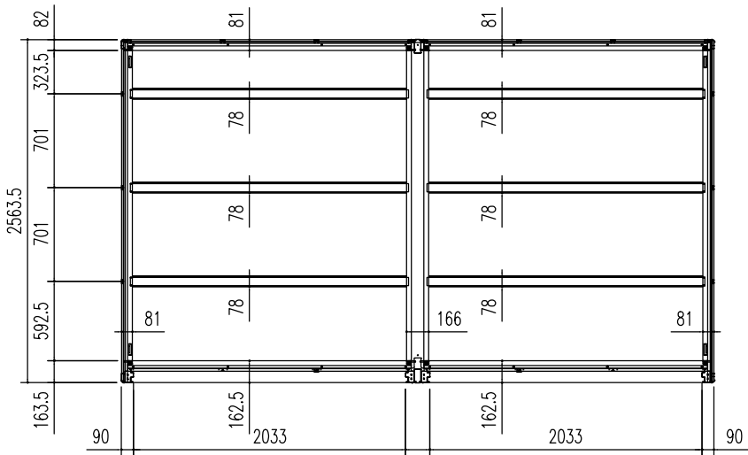
床伏図 (S=1/50)
