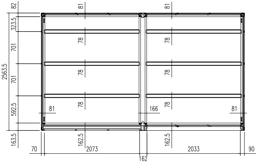
床伏図 (S=1/50)
