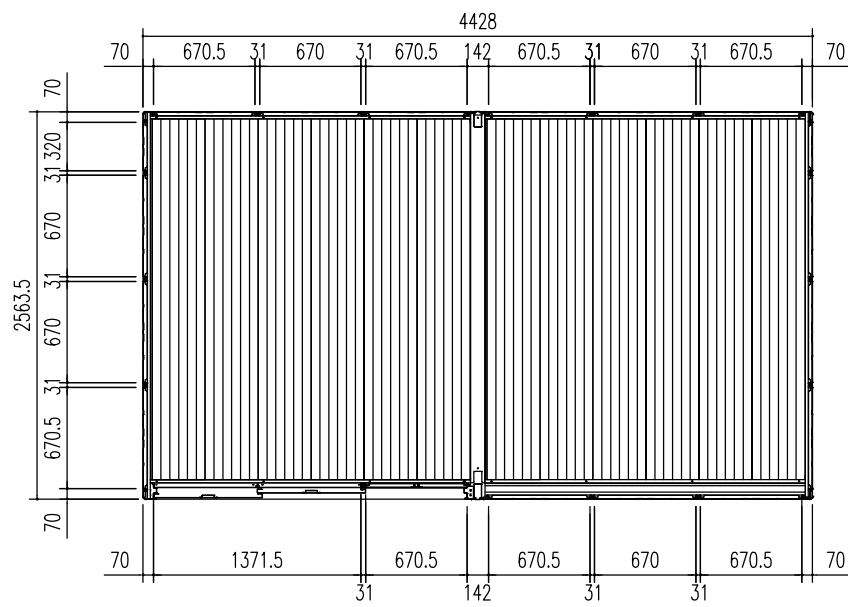
平面図 (S=1/50)
