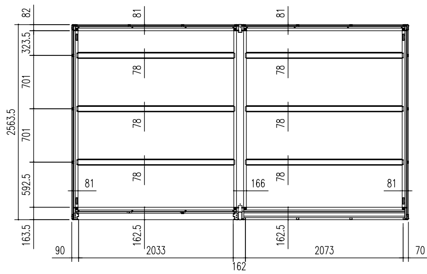
床伏図 (S=1/50)
