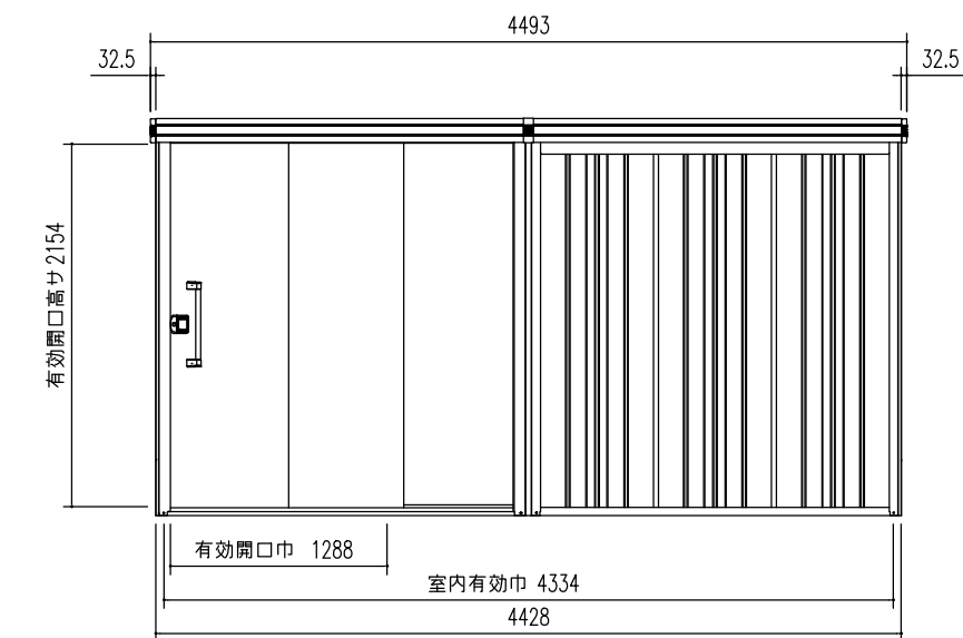
正面立面図 (S=1/50)
