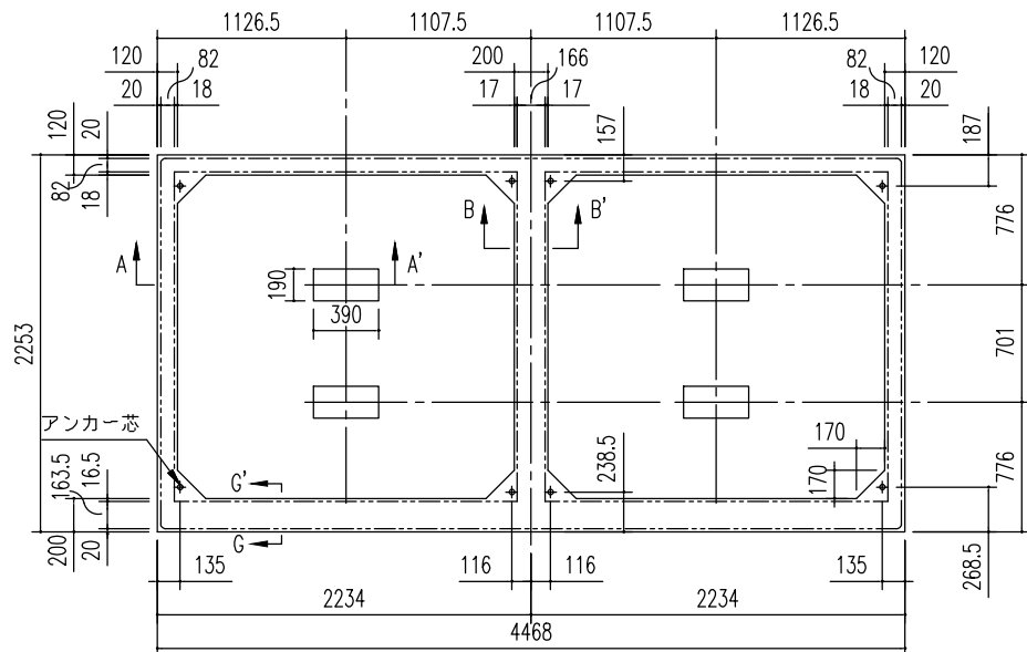
入口側 布基礎伏図 (S = 1/50)
