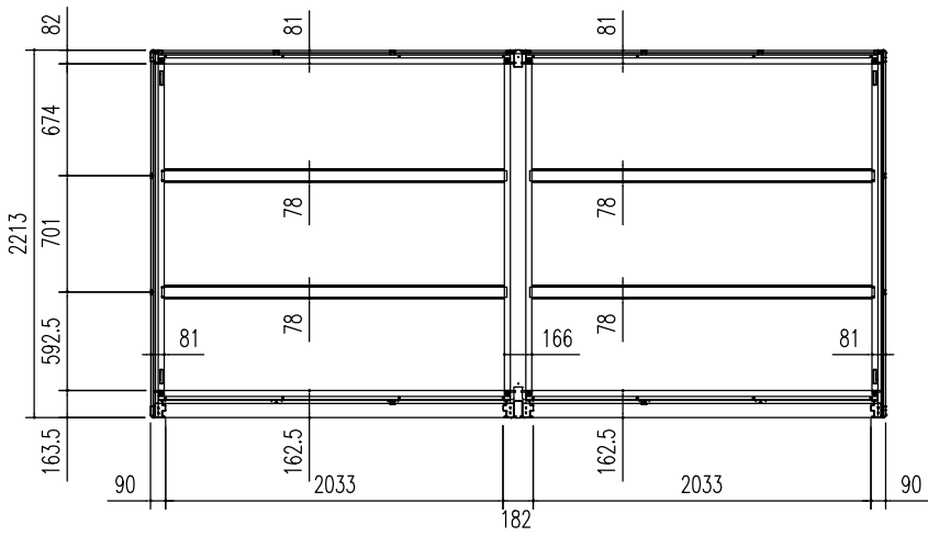
床伏図 (S=1/50)
