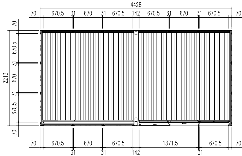
平面図 (S=1/50)
