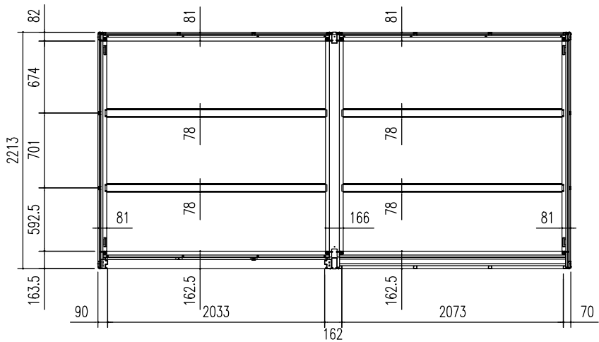
床伏図 (S=1/50)
