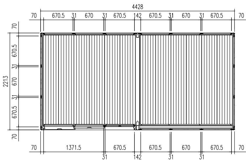
平面図 (S=1/50)
