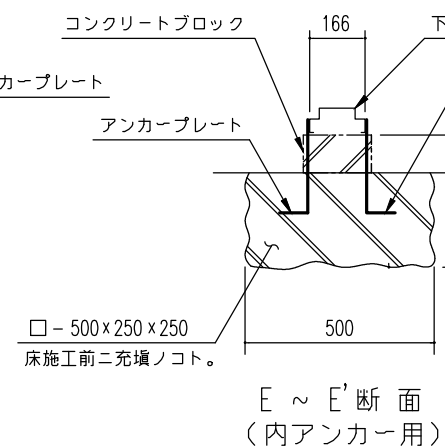
ブロック基礎断面図例 (S=1/20)
