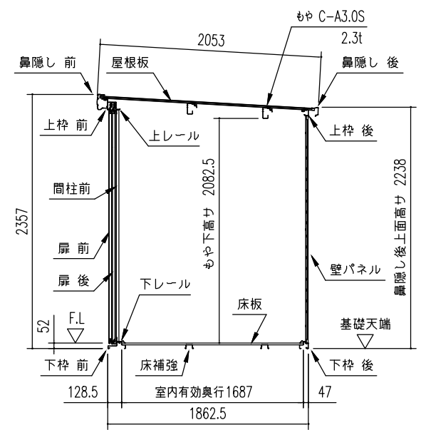
積雪型矩計図 (S=1/50)
