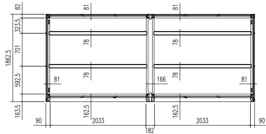
床伏図 (S= 1/50)
