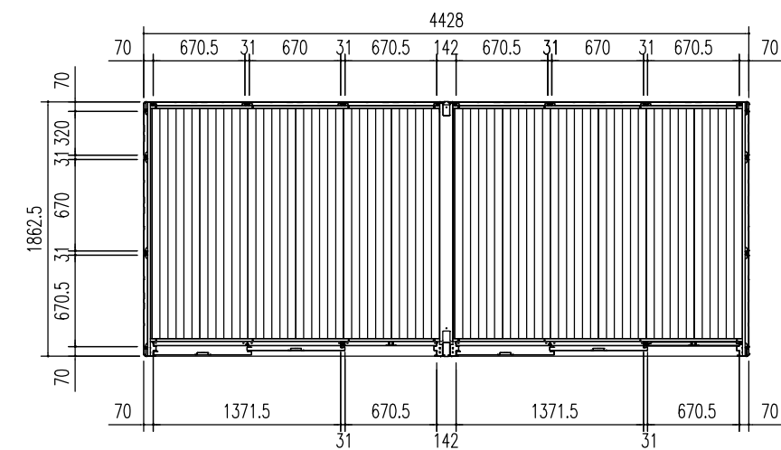
平面図 (S= 1/50)
