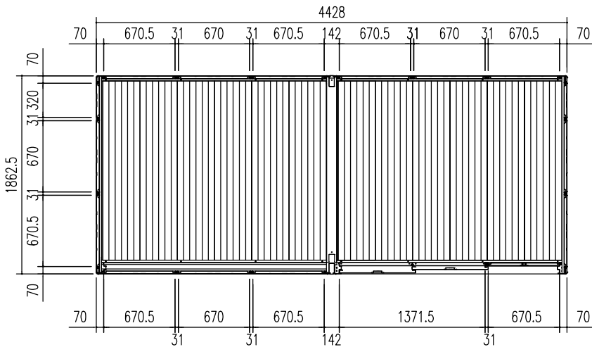
平面図 (S=1/50)
