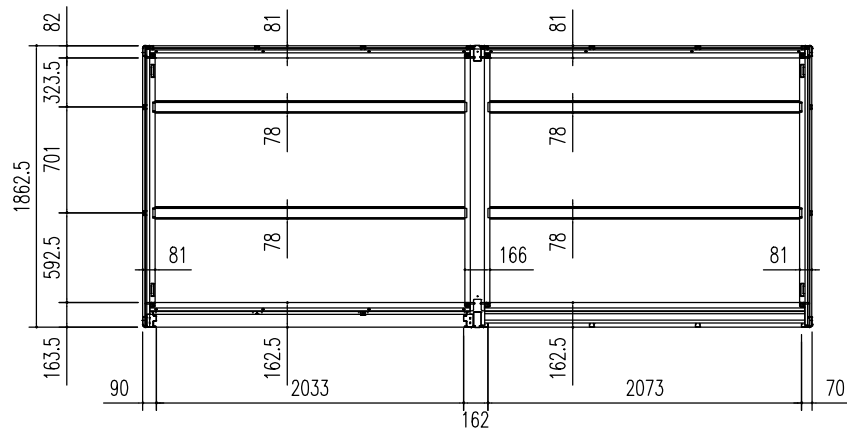
床伏図 (S=1/50)
