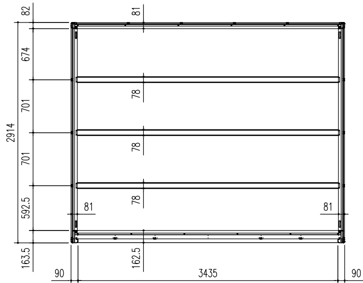
床 伏 図 (S = 1/50)
