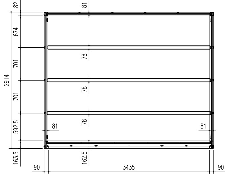
床伏図 (S = 1/50)
